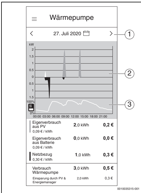
Bild 42 Wärmepumpe
