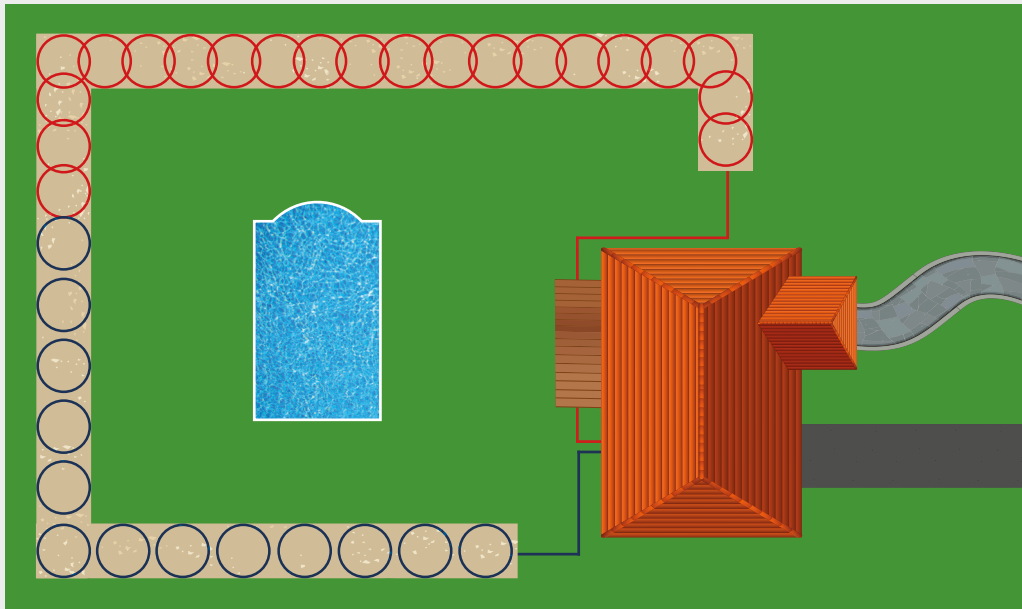
Ringgrabenkollektor
